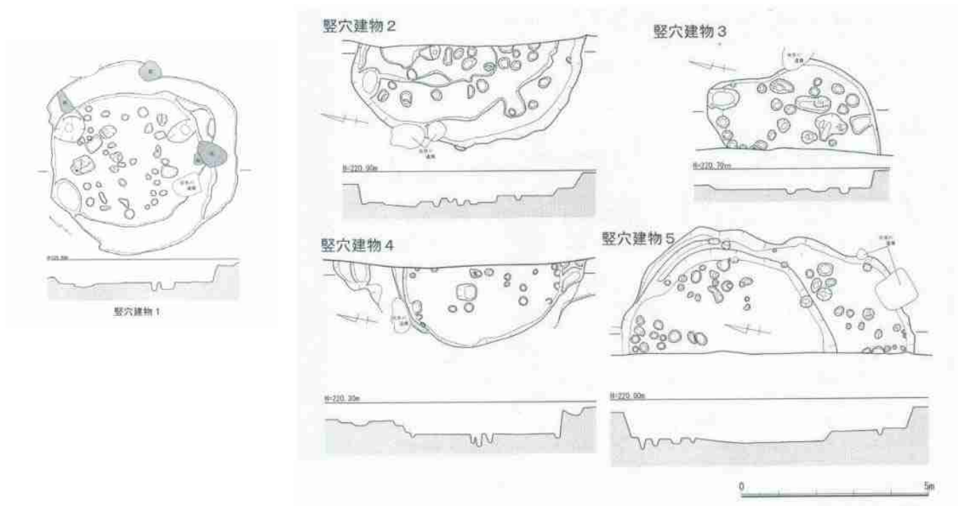
出土した縄文の竖穴式住居の平面図・立面図 現地説明資料より
