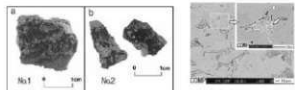
写真2 カマン・カレホック第IIIc層 鉄塊遺構出土鉄片の外觀。
