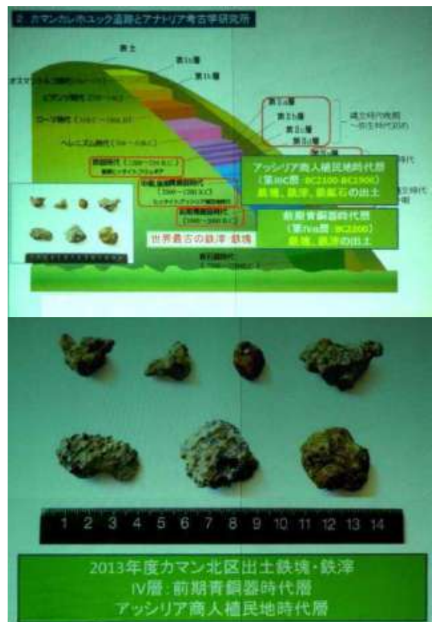
2013年カマン・カレホック遺跡の発掘調査で出土した ヒッタイト以前世界最古級の鉄滓と鉄滓 「古代ユーラシア大陸のアイアン ロード」研究報告
