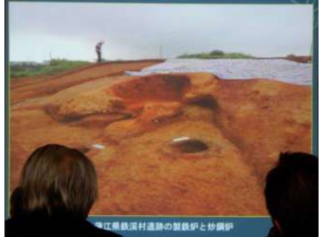
◎ 炉壁には石が用いられ、石の継ぎ目には耐火粘土が塗られ、炉内や周辺から大量の鉄滓、鉄鉱石、木炭が見つかった。
