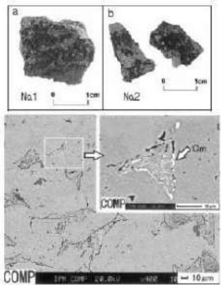
写真3 カマン・カレホユック遺跡第IIIc層出土No.1鉄片のEPMAによる組成像 (COMP)。Cmはセメントイト (Fe 3 C)。写真右上は枠内部を拡大。
