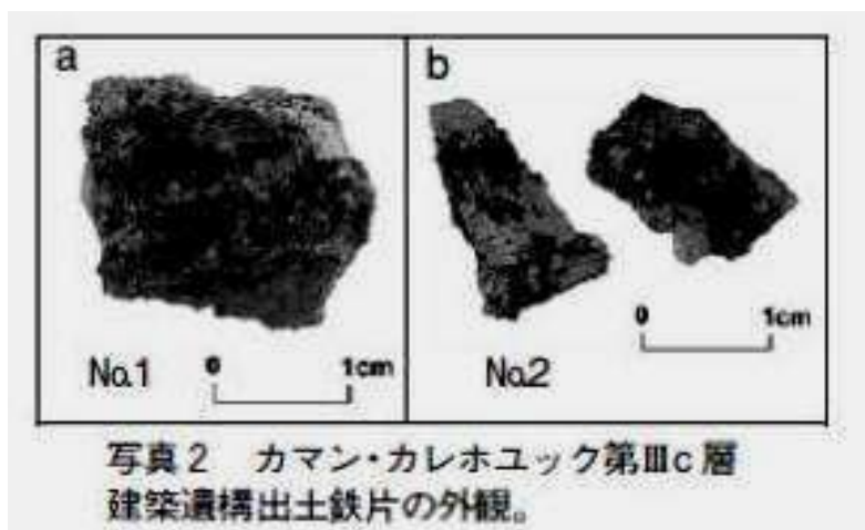
カマン・カレホユック遺跡の遺丘 BC19 世紀の層から出土した ヒッタイトの「鋼」
