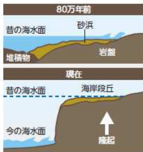
イメージ 海岸段丘の成り立ち
