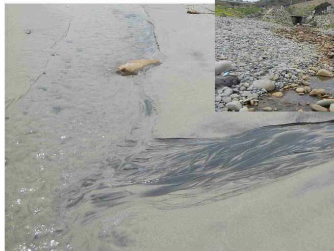
浜に堆積した砂鉄が描く文様 種子島 鉄浜海岸で 2013.4.16.
