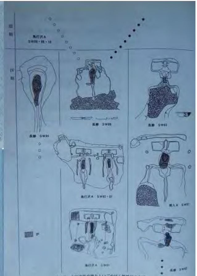
第15図 金沢地区の踏みふいご付製鉄炉の変遷
