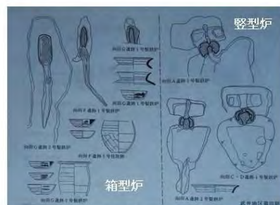
第Ⅲ期 箱型炉と踏み鞆のついた竪型炉出現の時代 8世紀中葉
