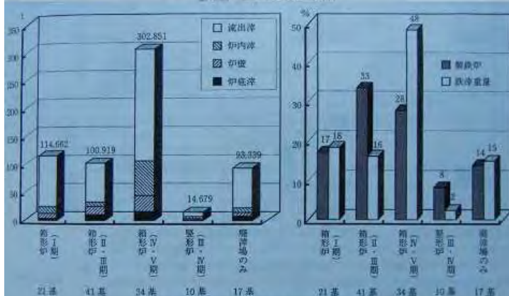
第14図 金沢地区製鉄炉廃滓量の推移
