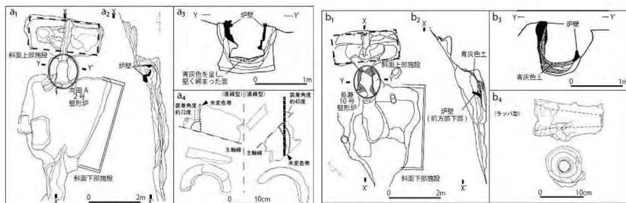
武井・金沢両製鉄遺跡群出土竪型炉と出土羽口の実測図
