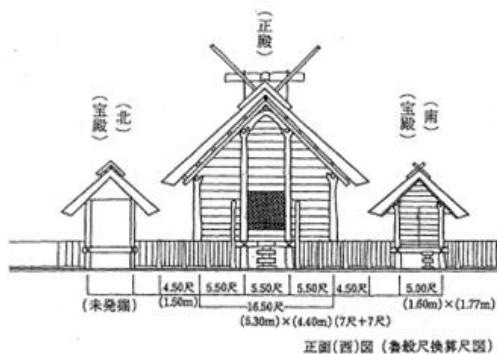
図7 太田地区検出の特殊建物復元案 (第20次)
