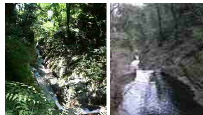
布引断層で地形がコの字に折れ曲がる布引溪谷
