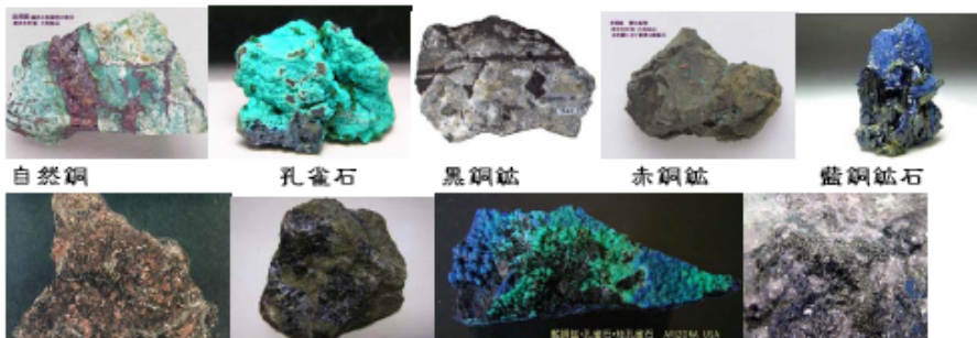
自然銅 孔雀石 黒銅鉱 赤銅鉱 藍銅鉱石 灰鉄輝石・赤銅鉱 灰鉄輝石・斑銅鉱 藍銅鉱・孔雀石・柱孔雀意思 輝銅鉱
